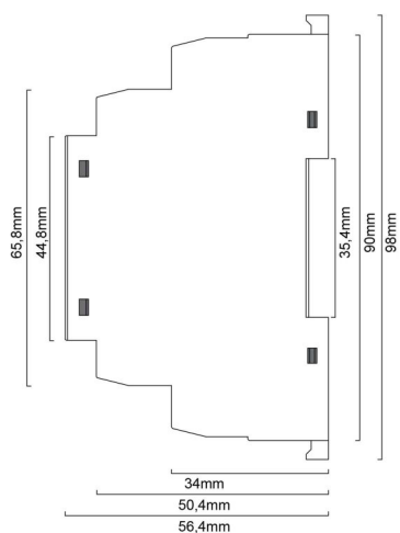
Geometrie Hutschiene
