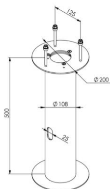
75.01574.03472 – Erdbodenhalter Beton-Anker HALM, STOCK, ALT, SCAN, OPP, EGER Mini
