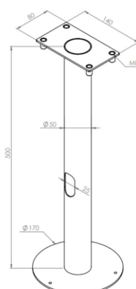
75.01555.03350 – Erdbodenhalter NAM
